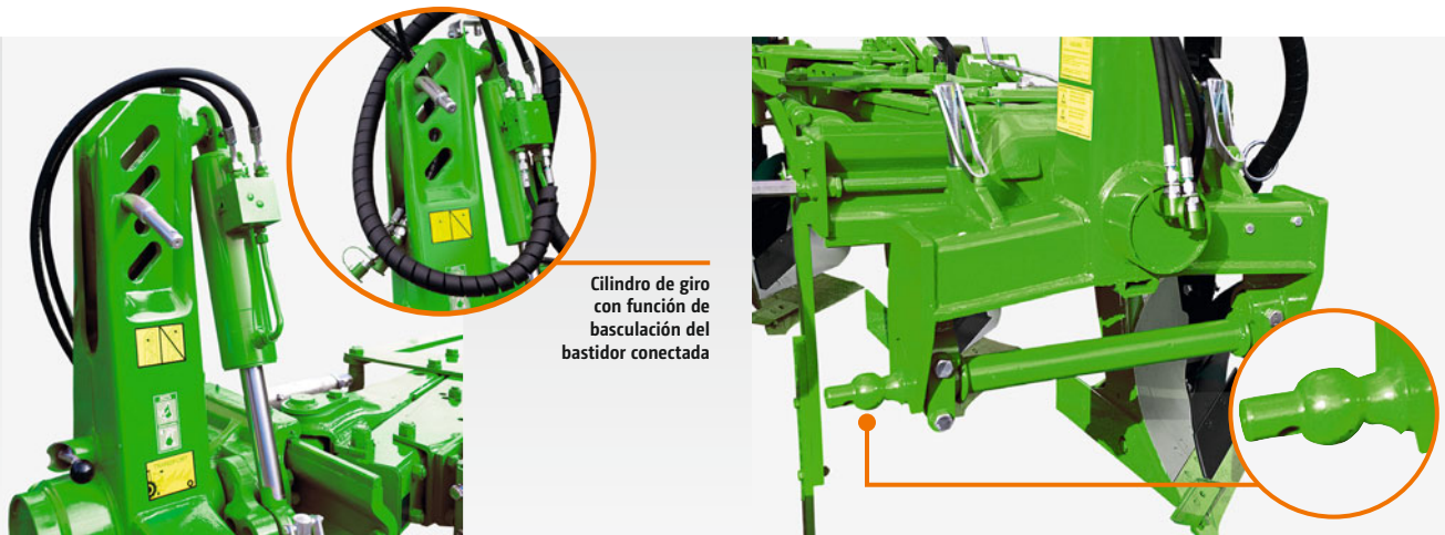
Cómodo sistema hidráulico de giro
