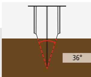
Suelo pesado Apoyo en los flancos
