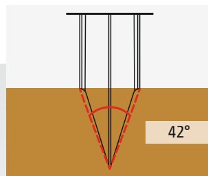
Suelo ligero Apoyo sobre el borde
